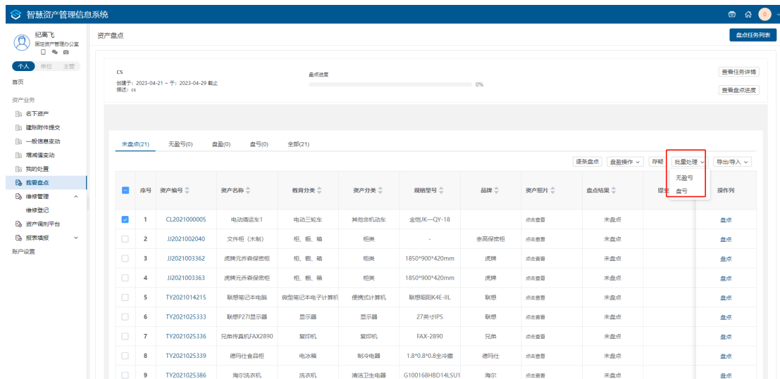
图30 批量处理
