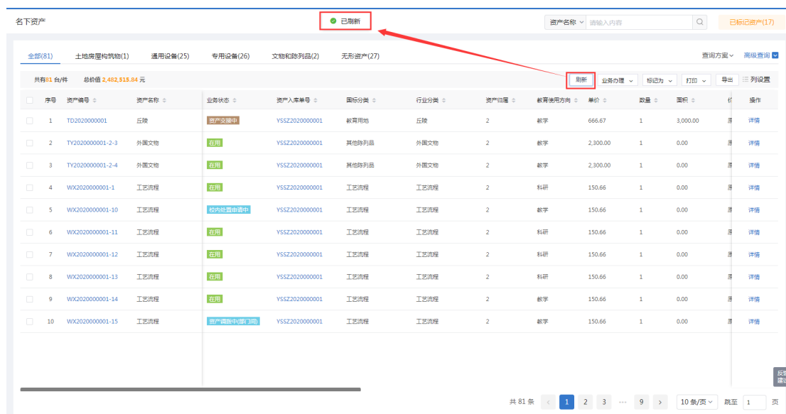
图6 刷新页面
