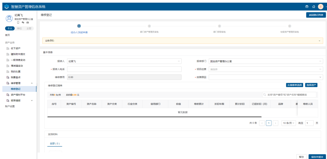
图15 登记申请单
