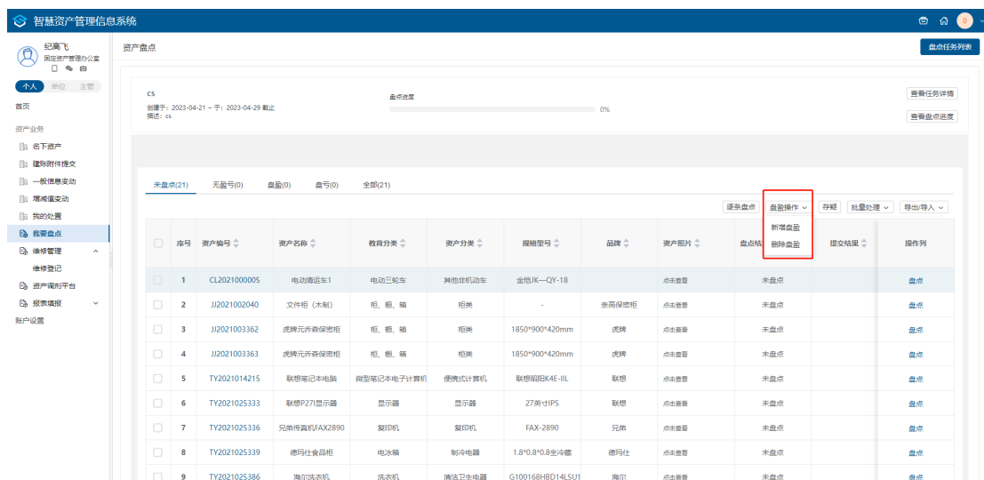
图28 盘点操作
